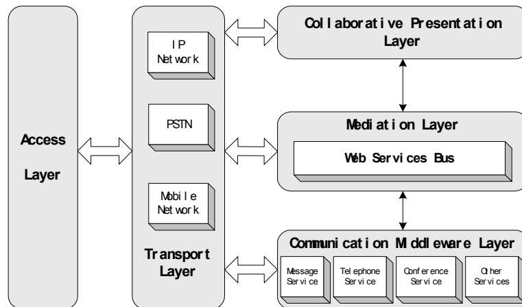
Fig. 2. WS-CSF Framework
